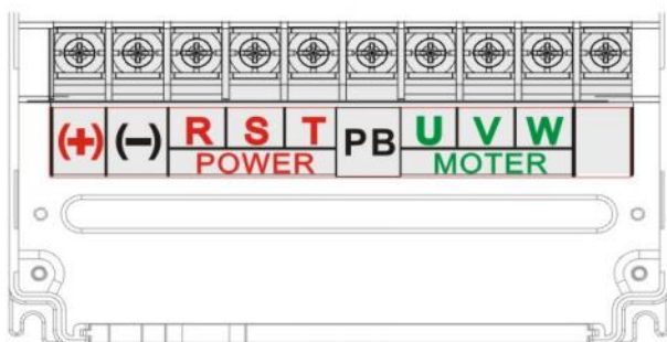
图3-8 三相380V(11-18.5KW)主回路端子图
