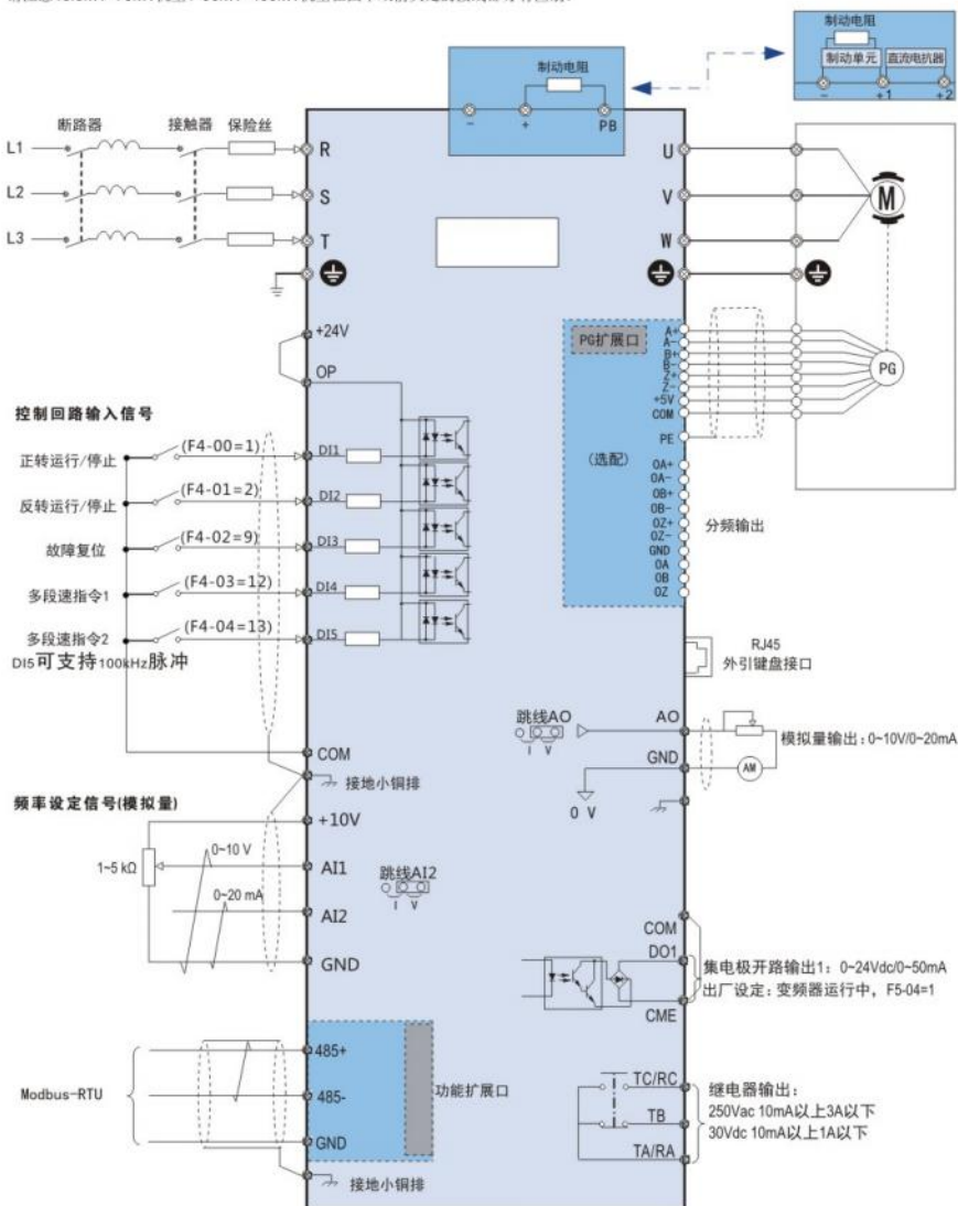
三相380V 典型接线图
