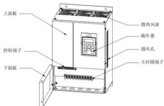
图2-3 22KW以上变频器部件名称
