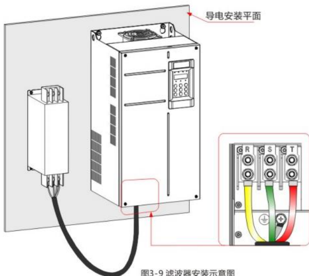
图3-9 滤波器安装示意图
