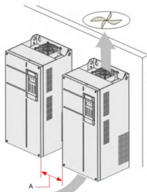
图3-3 多台变频器向上垂直安装
