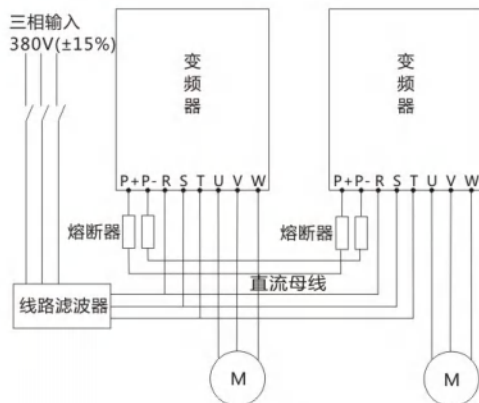
图3-12 共直流母线连接
