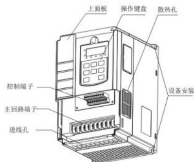
图2-2 18.5kW以下变频器部件名称
