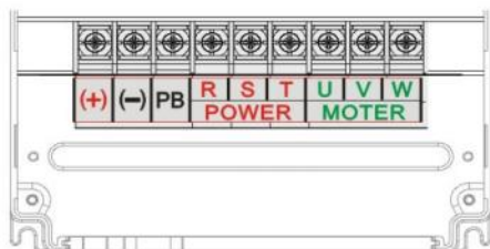
图3-7 三相380V(5.5-7.5KW)主回路端子分布图
