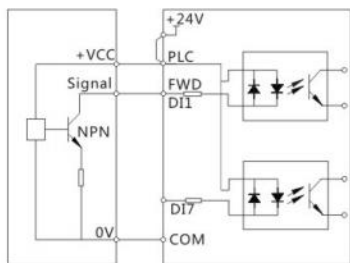
图3-15 NPN输入信号接线图
