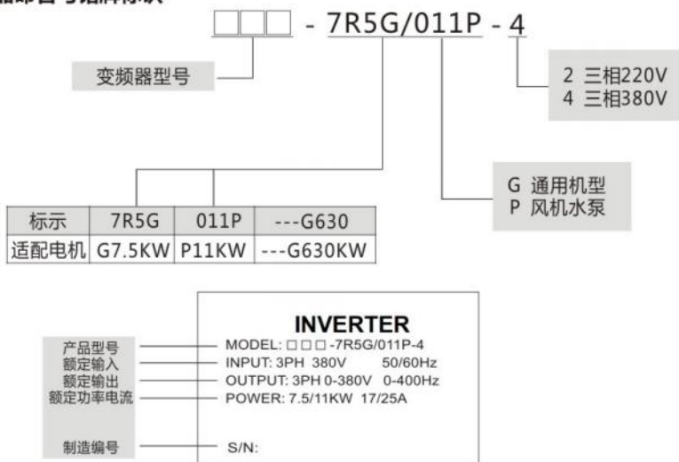
图2-1 产品命名与铭牌标识
