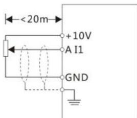
图3-13 模拟量端子接线图
