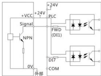
图3-17 NPN输入信号接线图
