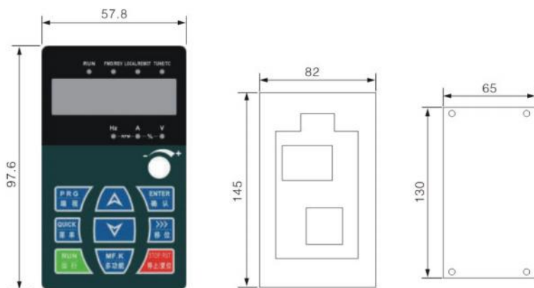
图2-6 键盘尺寸图
