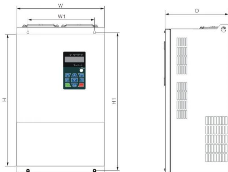
图2-8 变频器外型及安装尺寸
