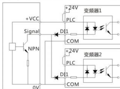
图3-19 多台变频器数字量并接接线图
