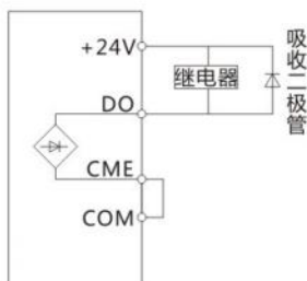
图3-20 使用内部24V接线图
