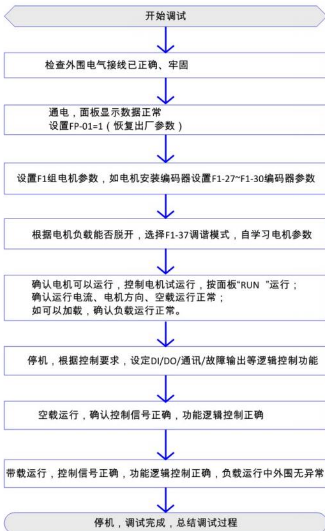
图4-3 快速调试步骤指南
