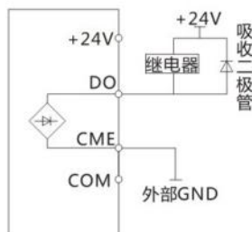
图3-21 使用外部24V接线图
