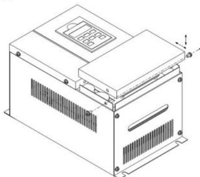
图3-4 盖板的安装与拆卸
