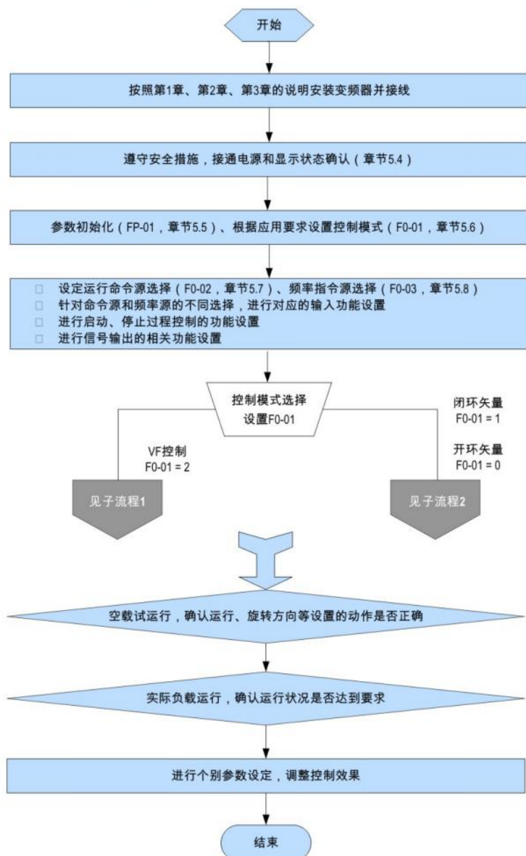
图4-4 变频器调试总流程图
