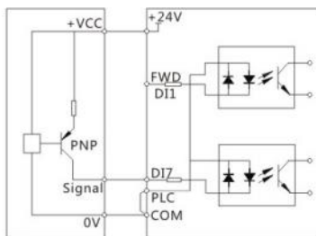
图3-16 PNP输入信号接线图
