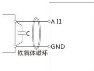
图3-14 模拟量端子处理图
