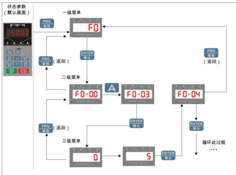
图4-2 三级菜单操作流程
