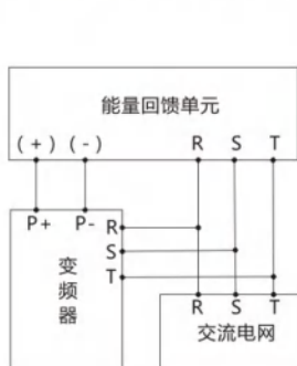
图3-11 能量回馈单元连接图
