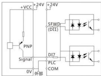
图3-18 PNP输入信号接线图
